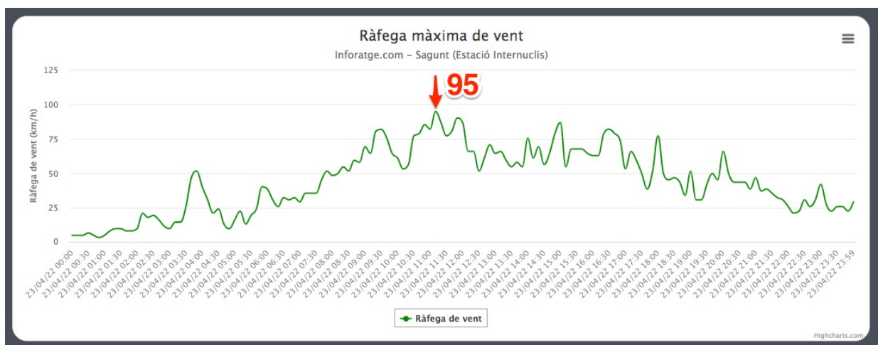
Ráfagas de viento registradas en SAGUNT (estación "Internuclis") el 13/08/22 (en km/h) https://inforatge.com/meteo-sagunt
