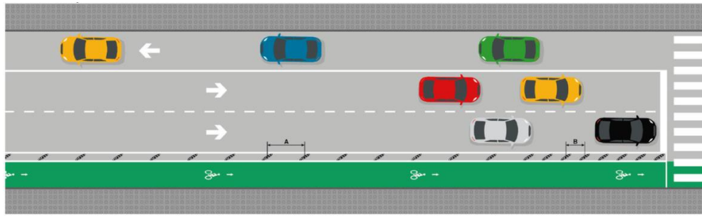
CONFIGURACIÓN EN OBLICUO A: 2600 mm (en el tramo). B: 1300 mm (en intersecciones).
