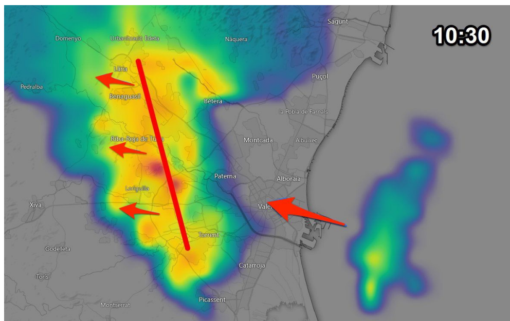
Imagen del radar correspondiente al sábado 12-11-2022 (10:30h)
