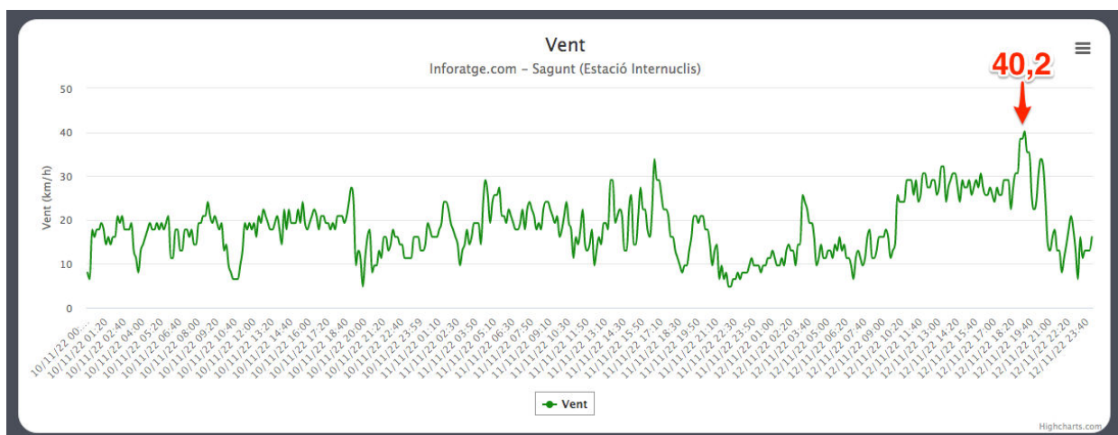
Ráfagas de viento registradas en SAGUNT (estación "Internuclis") entre el 10 y el 12/11/22 (en km/h) https://inforatge.com/meteo-sagunt
