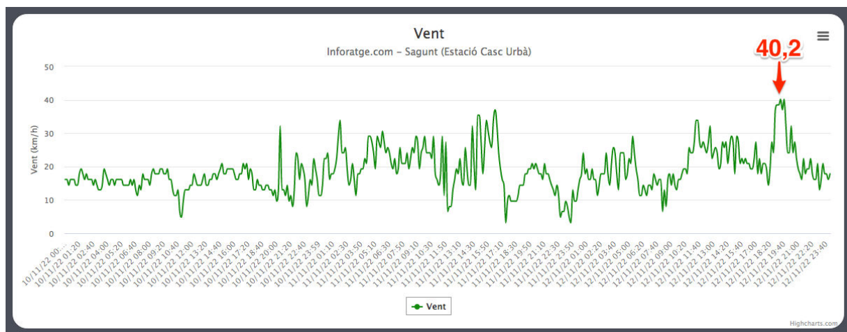
Ráfagas de viento registradas en SAGUNT (estación "Casc Urbà") entre el 10 y el 12/11/22 (en km/h) https://inforatge.com/meteo-sagunt
