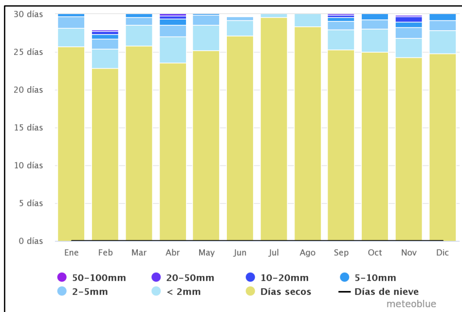
Il·lustració 6: quantitat de precipitació. Font:
