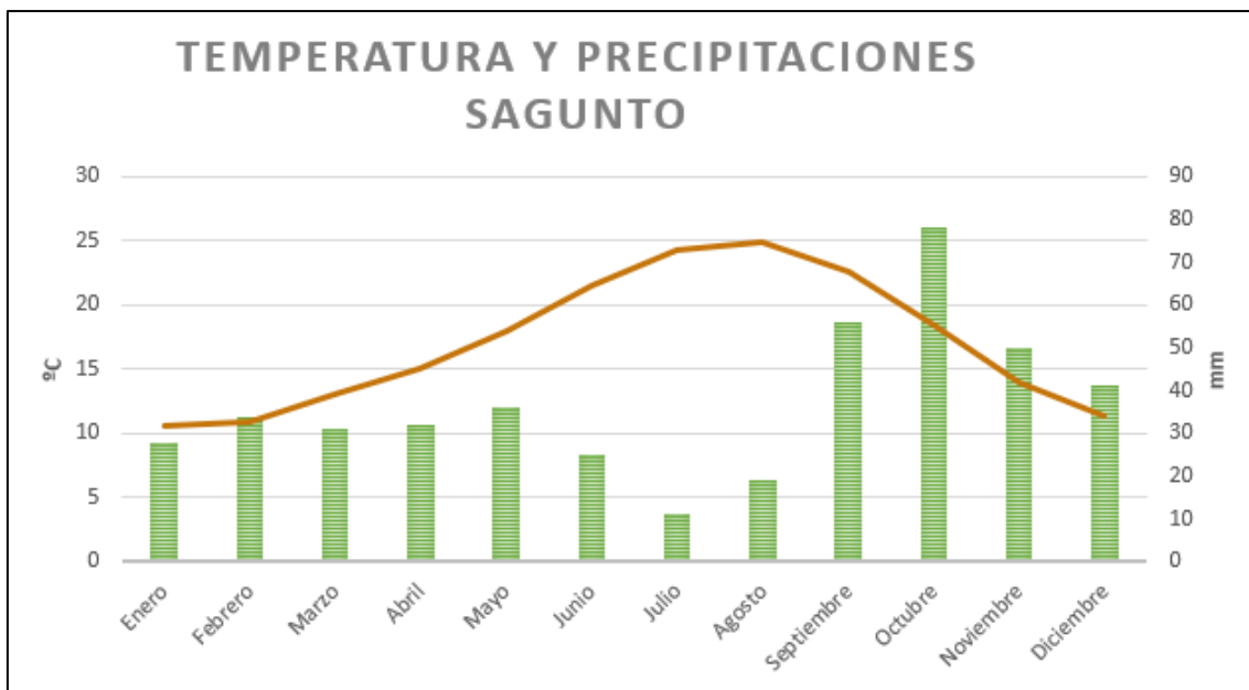
Il·lustració 5: climograma típic del municipi de Sagunt. Font: https://es.climate-data.org/europe/espana/comunidad-valenciana/sagunt-57166/
