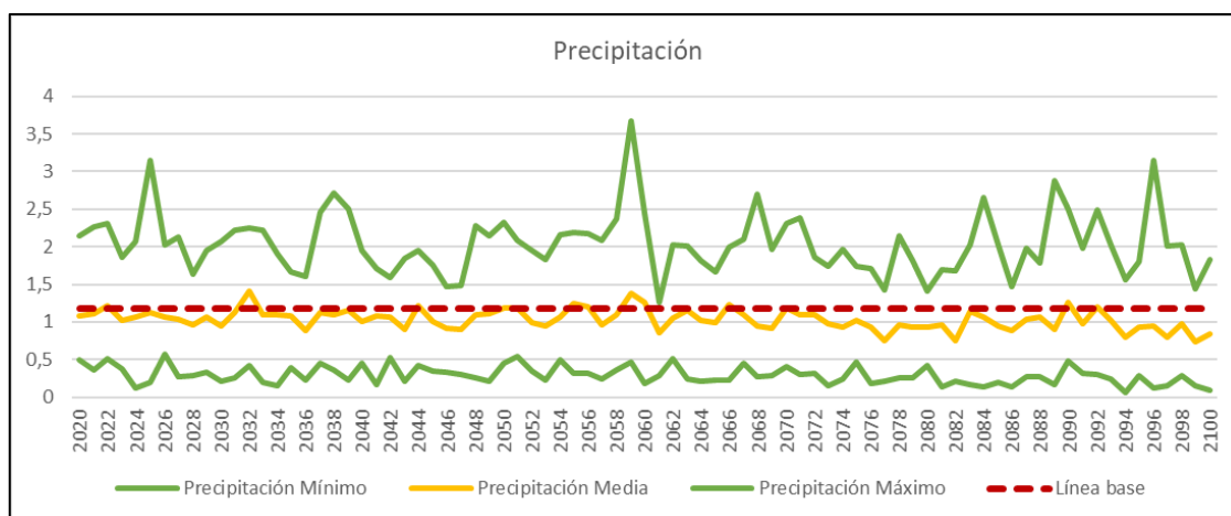
Gràfic 4: evolució de les precipitacions respecte de la línia base establida per a Sagunt. Font: https://www.adaptecca.es/
