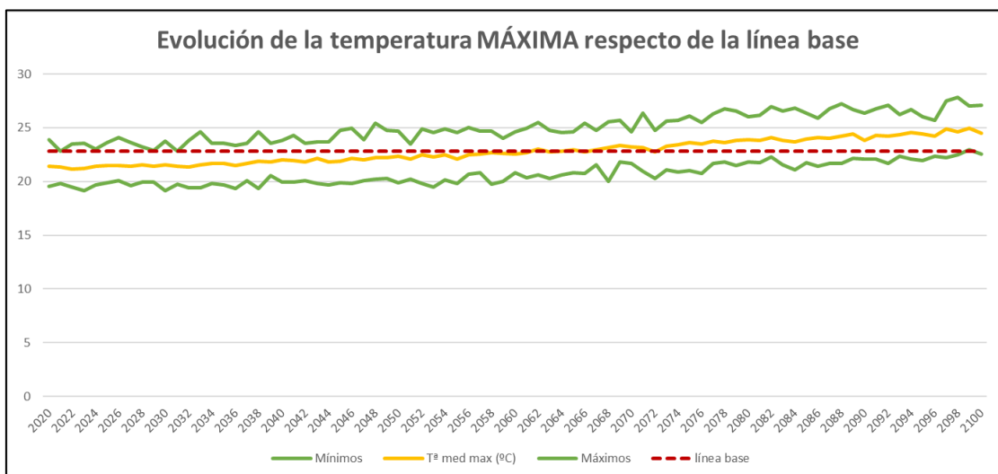
Gràfic 2: evolució de les temperatures màximes respecte de la línia base establida per a Sagunt. Font:
