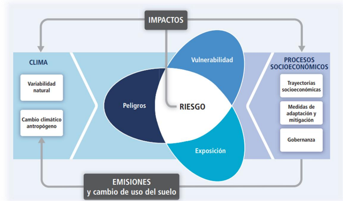
Il·lustració 5: il·lustració dels conceptes bàsics de la contribució del Grup de Treball II de l'IPCC.AR%. Resum tècnic.
