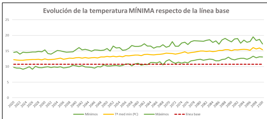
Gràfic 3: evolució de les temperatures mínimes respecte de la línia base establida per a Sagunt. Font:
