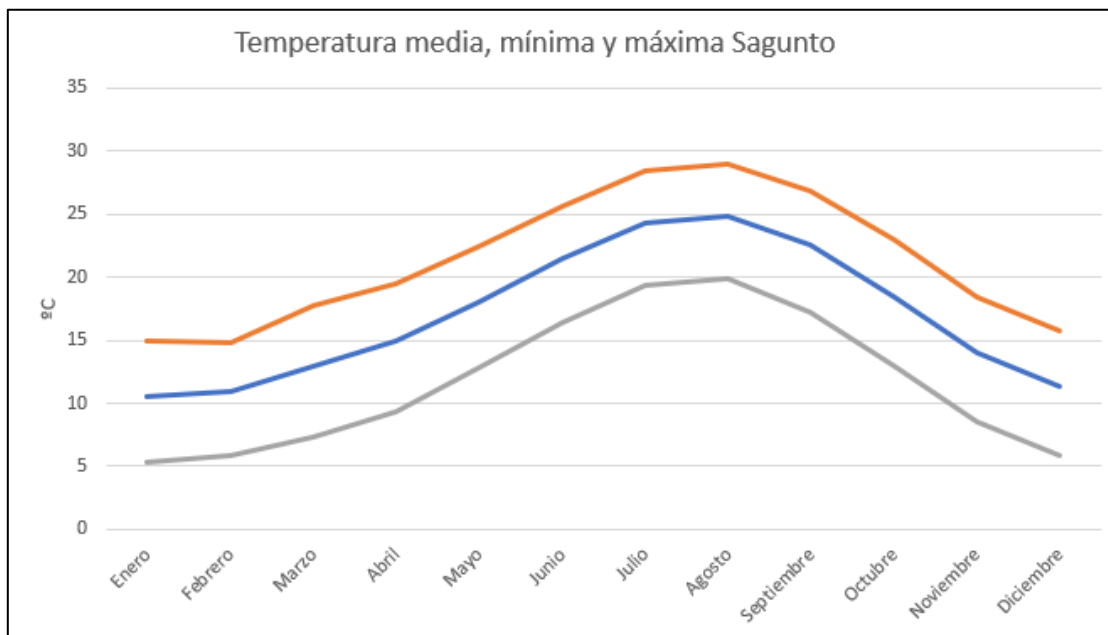
Il·lustració 4: diagrama de temperatura típic de Sagunt. Font: https://es.climate-data.org/europe/espana/comunidad-valenciana/sagunt-57166/
