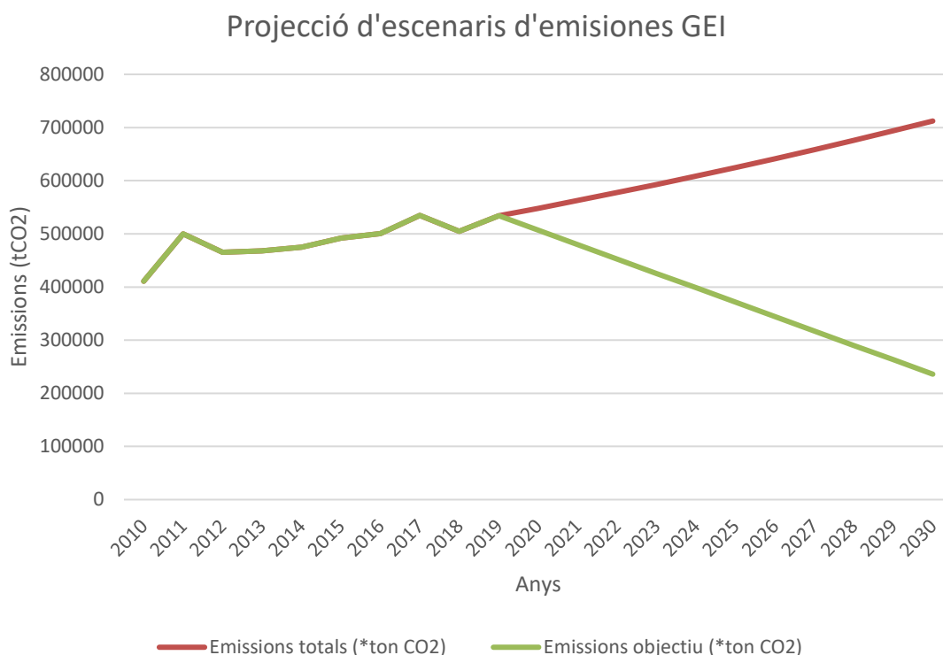
Gràfic 1: projeccions d'escenaris d'emissions de gasos amb efecte d'hivernacle al municipi de Sagunt.
