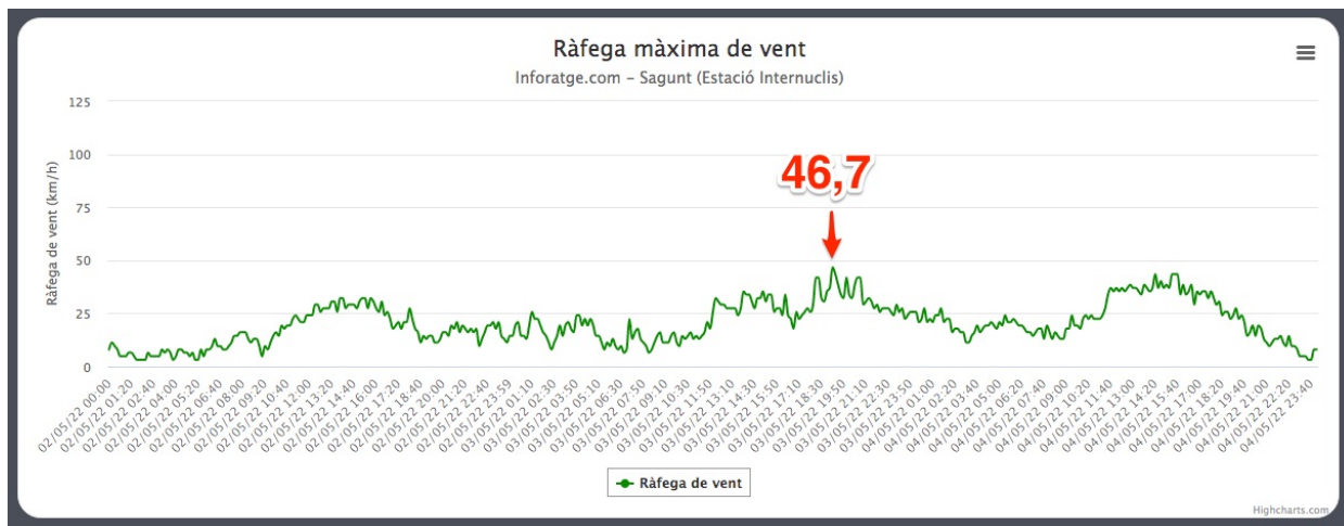
Ráfagas de viento registradas en SAGUNT (estación "Internuclis") el 03/05/22 (en km/h) https://inforatge.com/meteo-sagunt
