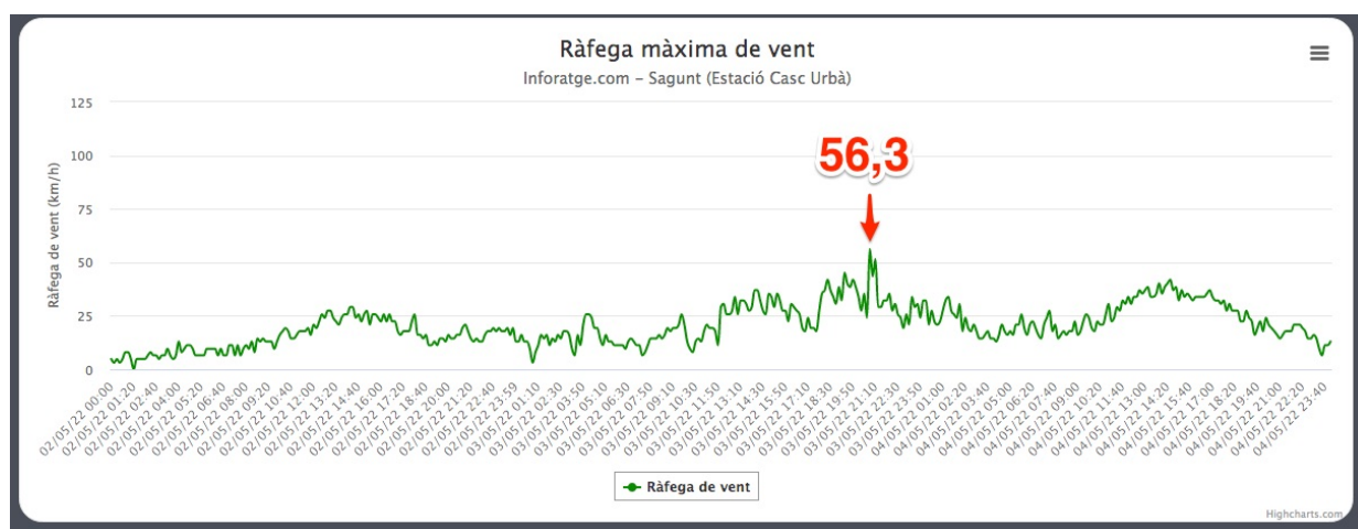
Ráfagas de viento registradas en SAGUNT (estación "Casc Urbà") el 03/05/22 (en km/h) https://inforatge.com/meteo-sagunt
